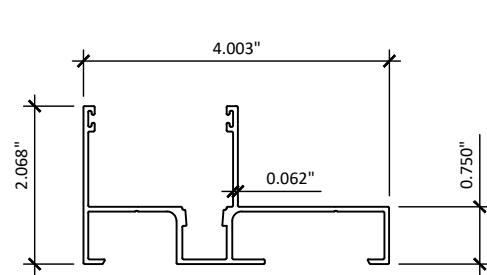
3 FRAME JAMB
