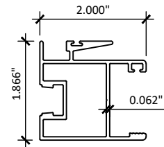
7 INTERLOCK STILE - EXTERIOR
